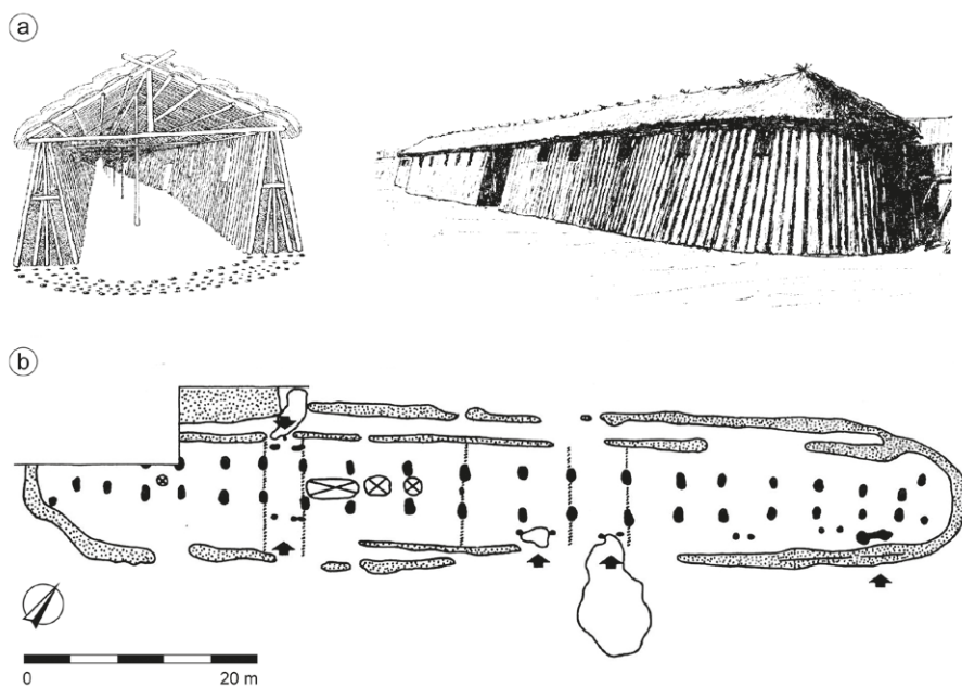
Obr. 4.1. Halové stavby: a – Kouřim (podle Šolle 1966); b – Borg (podle Šolle 1966, obr. 26–28, tab. XVII; Herschend – Kaldal Mikkelsen 2003, Fig. 1b).
