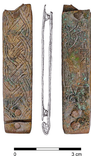
Obr. 5.7. Bodzia, stanoviště 1, okr. Włocławek. Bronzové opaskové nákončí z hrobu E864/I (viz obr. 5) s oboustrannou výzdobou, (stav po konzervaci): lící strana (foto z levé strany) s pletencem, rubová strana (foto z pravé strany) mj. s dvojzubcem Svatopluka I. Kyjevského, zvaného Prokletý. Strany jsou označeny v souladu s uložením předmětu v hrobě. Podle Beleckij 2018, s. 266, ris. 1.
