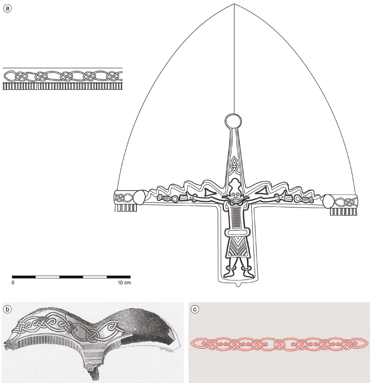
Obr. 4.2. Přilby: a – Svatováclavská přilba (kresba T. Vlasatý); b – nánosník z Lokrume na Gotlandu (podle Lindqvist 1925, 194, obr. 97, převzato z Vlasatý 2015); c – pletenec z přilby z Lokrume (podle Vlasatý 2015, kresba J. Zábránek). Za kresby a i c děkuji T. Vlasatému. K detailu lemu srov. Bravermanová et al. 2019, obr. 21.
