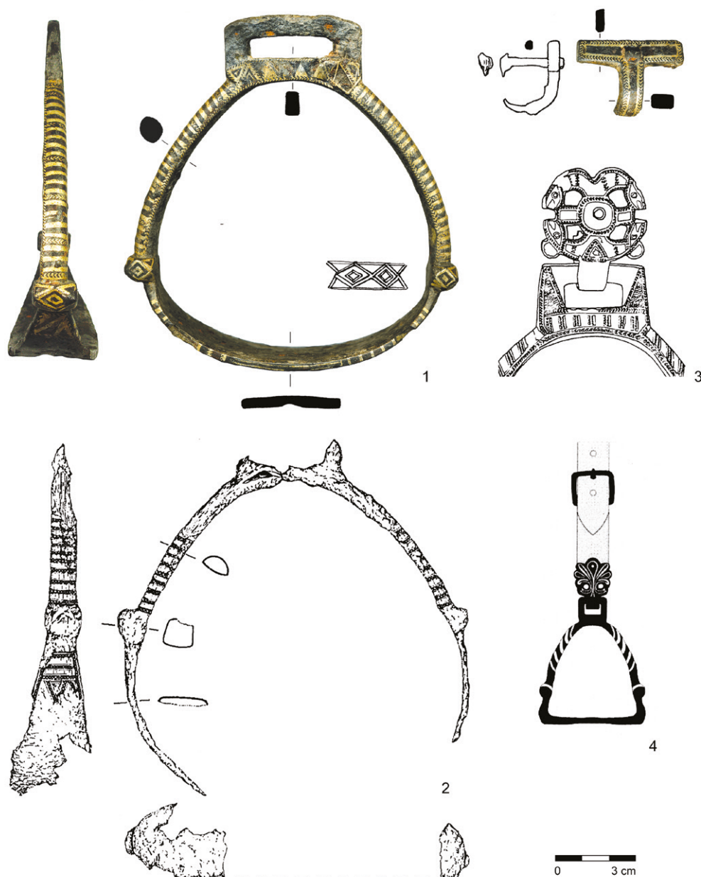
Obr. 4.5. 1 – Dobruška-Běstvíny, tausovaný třmen s průvlečkou, ovlivněný polskou produkcí či naopak ji inspirující. Konec 10. – 60. léta 11. století. Závěsná průvlečka se užívala v severském prostředí ke třmenům různých tvarů: 2 – Kalisz; 3 – Průtzke; 4 – Cieple. Podle Profantová 2012, Abb. 2, 5 (1, 2, 3); Wadyl 2019, ryc. 4: 30 (4).
