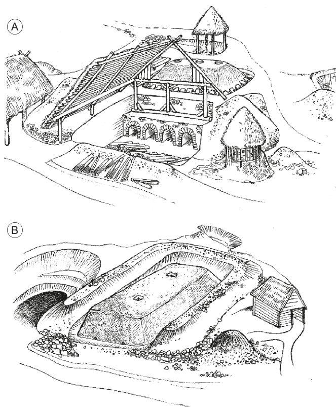
Obr. 13. Březina u Křtin. Volné rekonstrukce středověké kanálové vápenické pece (A) a raně novověkého milířiště (B). Kresba P. Kos.
