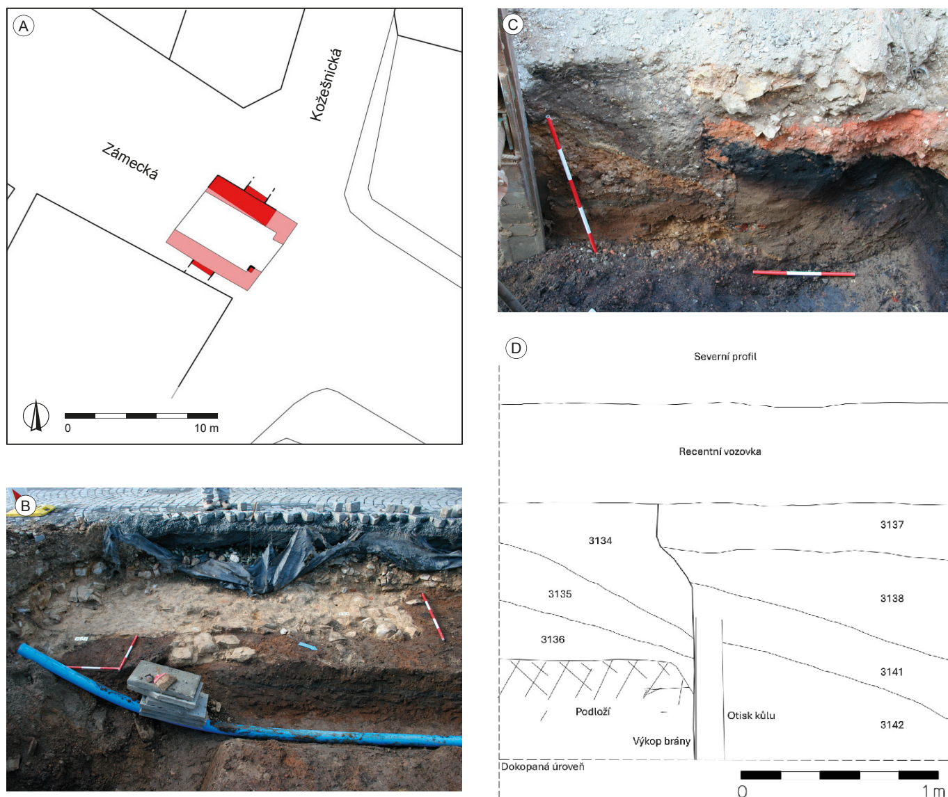
Obr. 3. Veselí nad Moravou, Horní brána. A – rekonstrukce půdorysné situace (tmavě červeně zachycené úseky, světle červeně předpokládané zdivo, čárkovaně hypotetický průběh hradby); B – severovýchodní nároží brány během výzkumu v roce 2011 v popředí relikv městské hradby narušené mladším výkopem (v místě severky); C – severní profil nově budované kanalizace v průjezdu původní brány; D – stejná situace na dokumentovaném řezu. Foto a kresba Archaia Brno z. ú.
