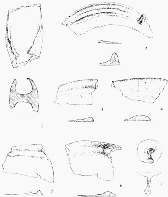
Obr. 2. Boskovice (okr. Blansko). „Pod Lipníky“ a „Panina louka“. Zlomky bronzových předmětů. Boskovice (Bez. Blansko). „Pod Lipníky“ u. „Panina louka“. Fragmente der Bronzegegenstände.
