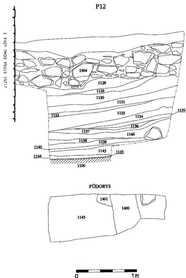
Obr. 10. Čajkovského 34-36, Úzká 3. Řez zásypu suterénu dřevohlíněného domu. Čajkovského Strasse Nr. 34-36, Úzká Strasse Nr. 3. Schnitt durch das Souterrain des Holz-Erde-Hauses.
